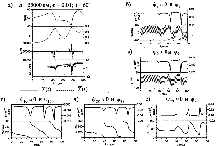
Рисунок 6 — Орбитальная динамика объекта под действием наложения большого числа вековых резонансов с различным характером изменения критических аргументов. а) долговременная орбитальная эволюцию элементов орбиты и параметров MEGNO; б) – е) изменение во времени резонансных соотношений вековых резонансов и их критических аргументов
