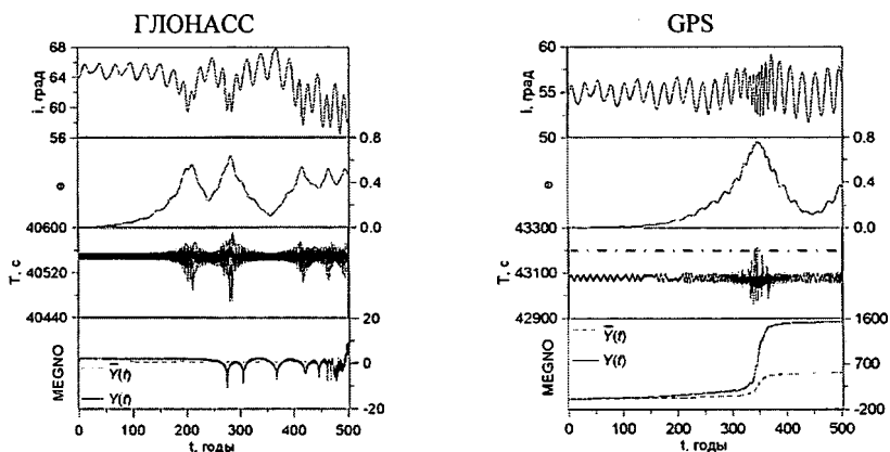
Рисунок 1 — Эволюция наклона i , эксцентриситета e , периода T и параметров MEGNO (неосредненный параметр Y(t) — сплошная линия и осредненный \bar{Y}(t) — пунктирная линия) для объектов ГЛОНАСС и GPS на орбитах функционирования
